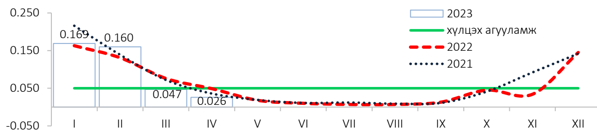
ЗУРАГ 4. УЛААНБААТАР 4 ХОТЫН АГААР ДАХЬ ХҮХЭРЛЭГ ХИЙН АГУУЛАМЖ, 13 СТАНЦЫН ДУНДАЖ, мг/м 3
