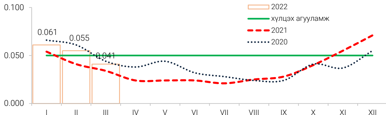
Зураг 6. Улаанбаатар 4 хотын агаар дахь 10 микроноос бага хэмжээтэй тоосны агууламж, 12 станцын дундаж, мг/м 3
