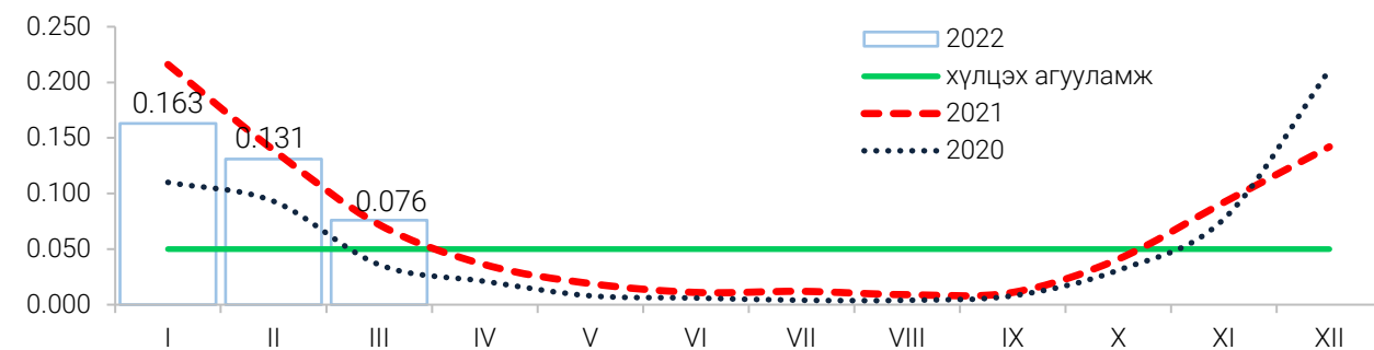
Зураг 5. Улаанбаатар 4 хотын агаар дахь азотын давхар ислийн агууламж, 10 станцын дундаж, мг/м 3
