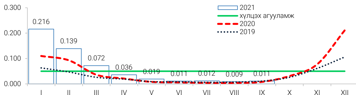
Зураг 5. Улаанбаатар 3 хотын агаар дахь азотын давхар ислийн агууламж, 11 станцын дундаж, мг/м 3
