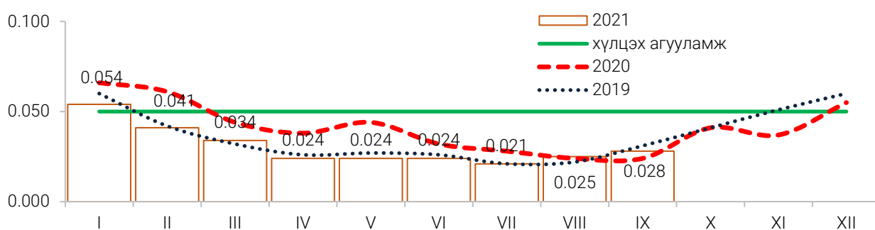
Зураг 6. Улаанбаатар 3 хотын агаар дахь 10 микроноос бага хэмжээтэй тоосны агууламж, 12 станцын дундаж, мг/м 3
