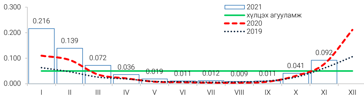
Зураг 5. Улаанбаатар 3 хотын агаар дахь азотын давхар ислийн агууламж, 11 станцын дундаж, мг/м 3
