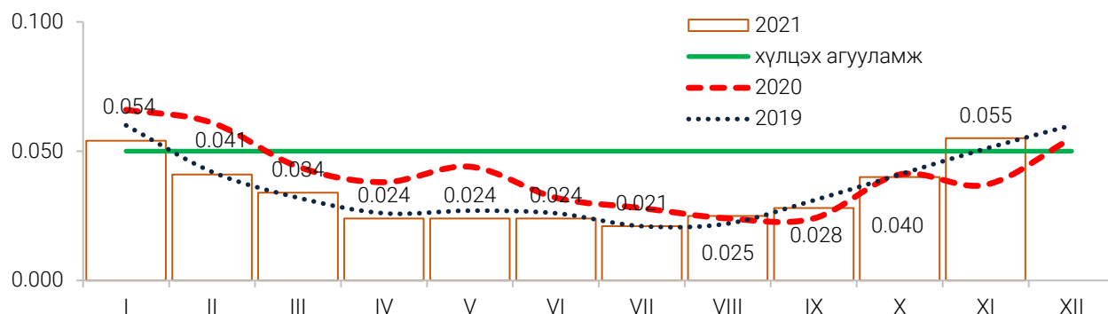
Зураг 6. Улаанбаатар 3 хотын агаар дахь 10 микроноос бага хэмжээтэй тоосны агууламж, 12 станцын дундаж, мг/м 3
