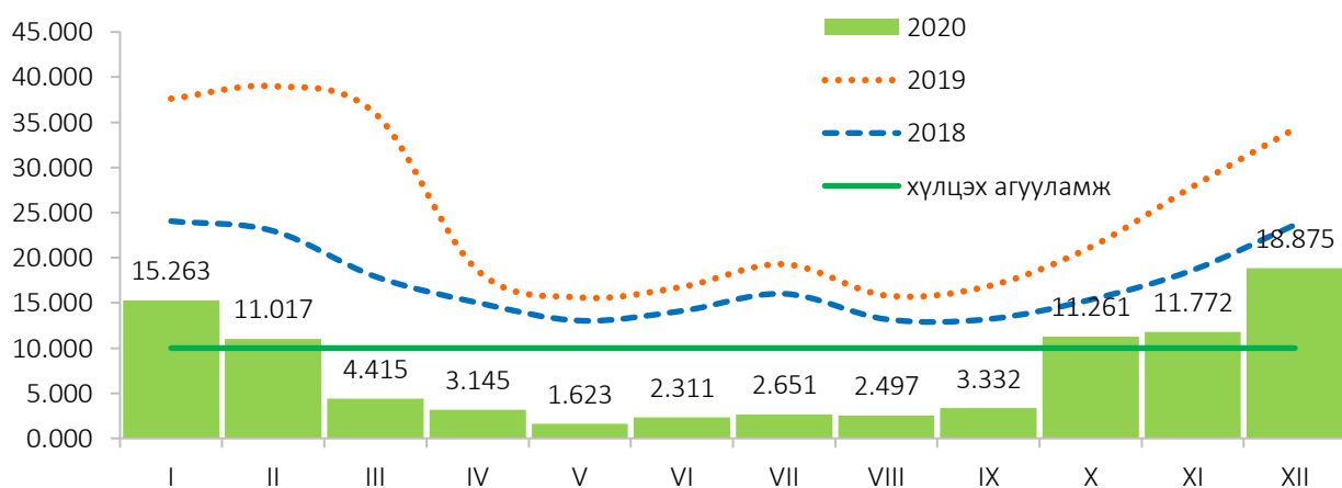
Зураг 14. Улаанбаатар 3 хотын агаар дахь нүүрстөрөгчийн дутуу исэл, 17 харуулын дундаж, сараар, мг/м 3
