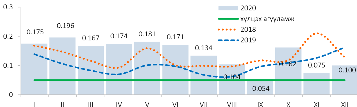
Зураг 13. Улаанбаатар 3 хотын агаар дахь азотын давхар ислийн агууламж, 17 харуулын дундаж, сараар, мг/м 3
