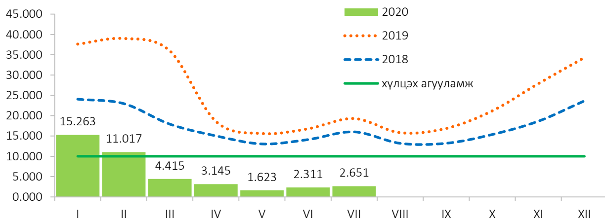
Зураг 14. Улаанбаатар 3 хотын агаар дахь нүүрстөрөгчийн дутуу исэл, 15 харуулын дундаж, сараар, мг/м 3
