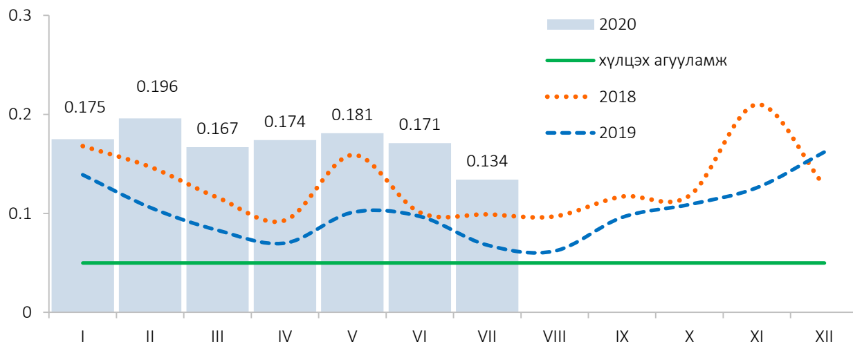
Зураг 14. Улаанбаатар 3 хотын агаар дахь нүүрстөрөгчийн дутуу исэл, 15 харуулын дундаж, сараар, мг/м 3
