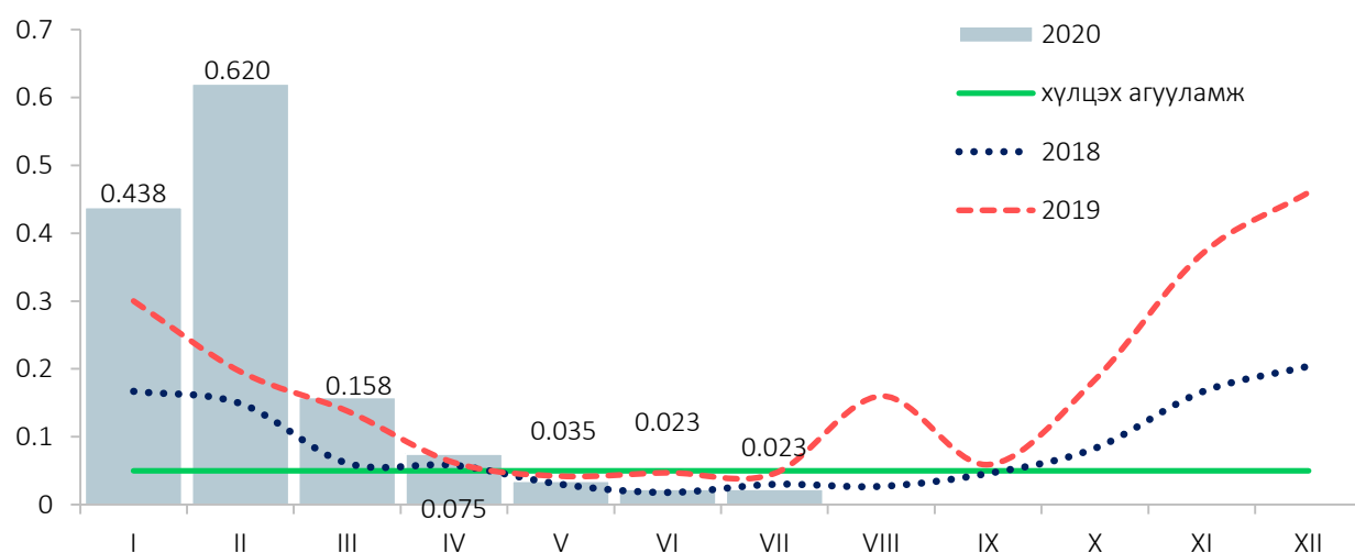
Зураг 12. Улаанбаатар 3 хотын агаар дахь хүхэрлэг хийн агууламж, 15 харуулын дундаж, сараар, \text{мг}/\text{м}^3
