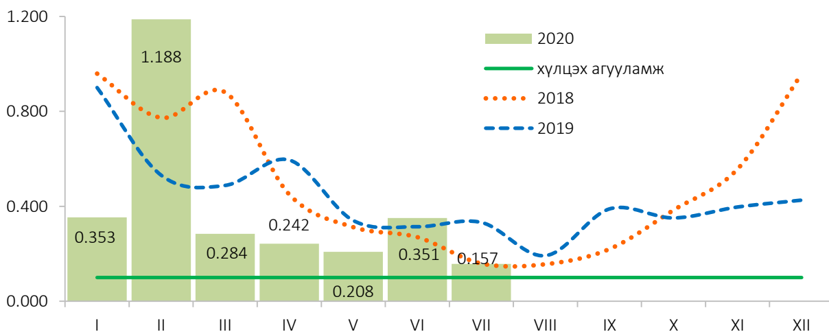
Зураг 15. Улаанбаатар 3 хотын агаар дахь 10 микроноос бага хэмжээтэй тоосны агууламж, 15 харуулын дундаж, сараар, мг/м 3
