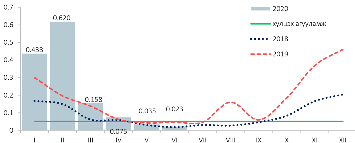
Зураг 12. Улаанбаатар 3 хотын агаар дахь хүхэрлэг хийн агууламж, 15 харуулын дундаж, сараар, мг/м 3
