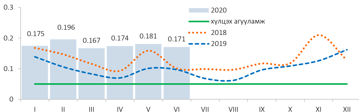
Зураг 14. Улаанбаатар 3 хотын агаар дахь нүүрстөрөгчийн дутуу исэл, 15 харуулын дундаж, сараар, мг/м 3
