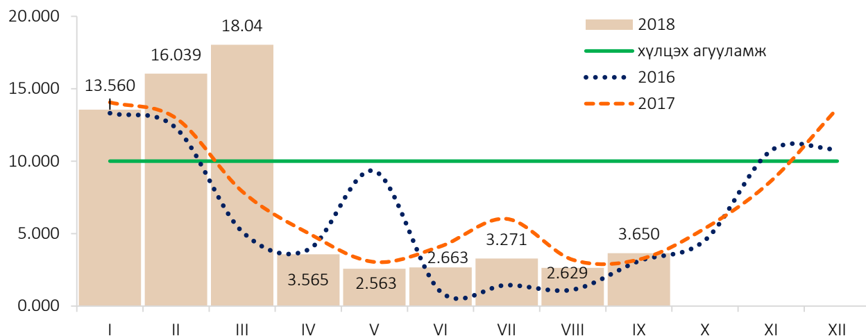
Зураг 9. Улаанбаатар 3 хотын агаар дахь нүүрстөрөгчийн дутуу исэл, 12 харуулын дундаж, сараар, мг/м 3
