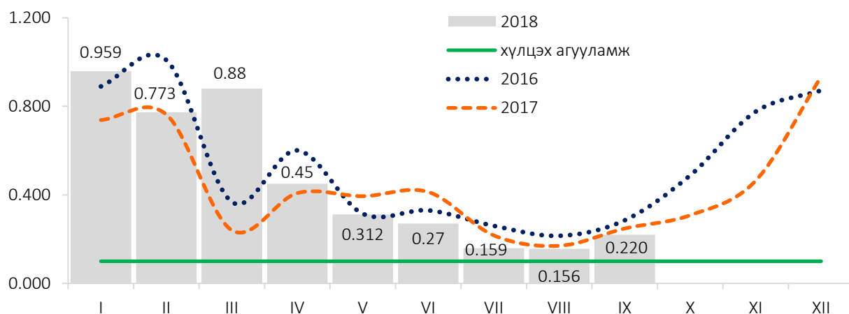
Зураг 10. Улаанбаатар 3 хотын агаар дахь 10 микроноос бага хэмжээтэй тоосны агууламж, 12 харуулын дундаж, сараар, мг/м 3
