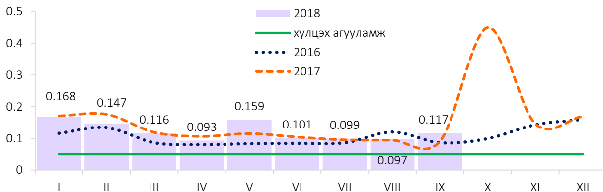
Зураг 9. Улаанбаатар 3 хотын агаар дахь нүүрстөрөгчийн дутуу исэл, 12 харуулын дундаж, сараар, мг/м 3
