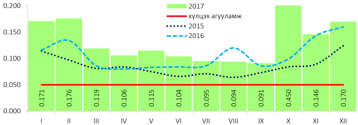
Зураг 53. Улаанбаатар 3 хотын агаар дахь нүүрстөрөгчийн дутуу исэл, 12 харуулын дундаж, сараар, мг/м 3
