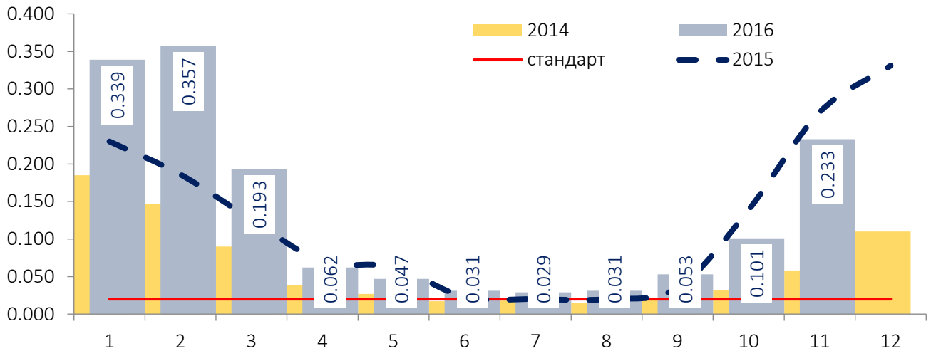
Зураг 24. Хүхэрлэг хийн агууламж, мг/м 3
