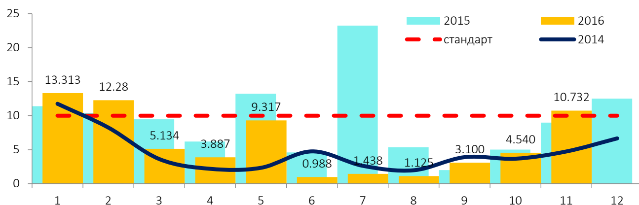
Зураг 27. Нүүрстөрөгчийн дутуу исэл, мг/м 3
